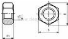
Piulita hex ISO TYP -1 TYP-2
