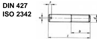
stift filet si slitz
